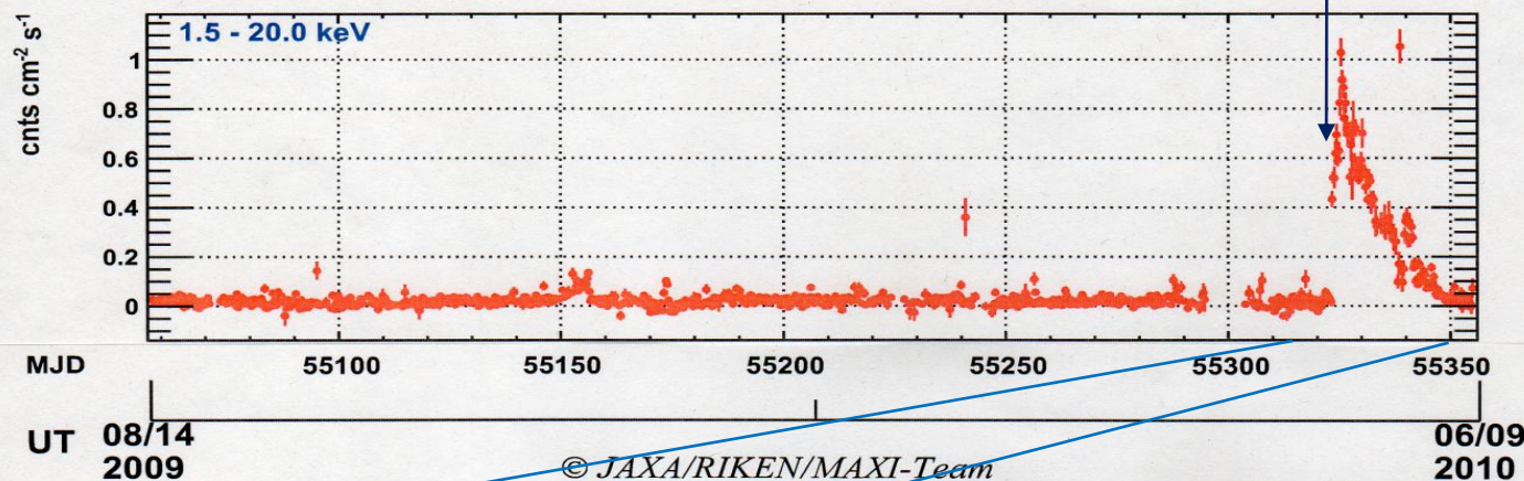
CirX-1 のX線強度曲線
